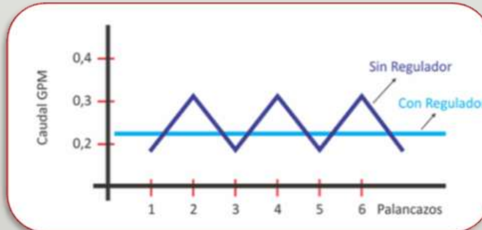
REGULADOR DE PRESIÓN 21 PSI REFERENCIA : R1116SY
